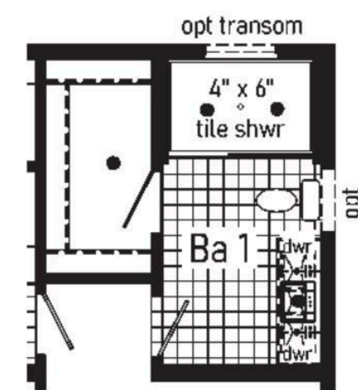
Optional 4'x6' Walk-In Shower Omits linen.
